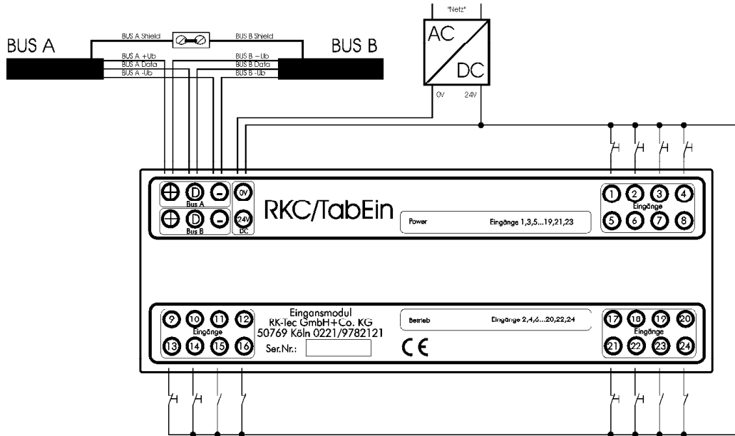
Abb. 1 - Beschaltung TabEin-Modul
