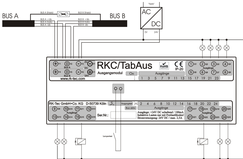
Abb. 2 - Beschaltung TabAus-Modul
